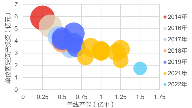
图 13：单线产能与单位投资额呈负相关关系
