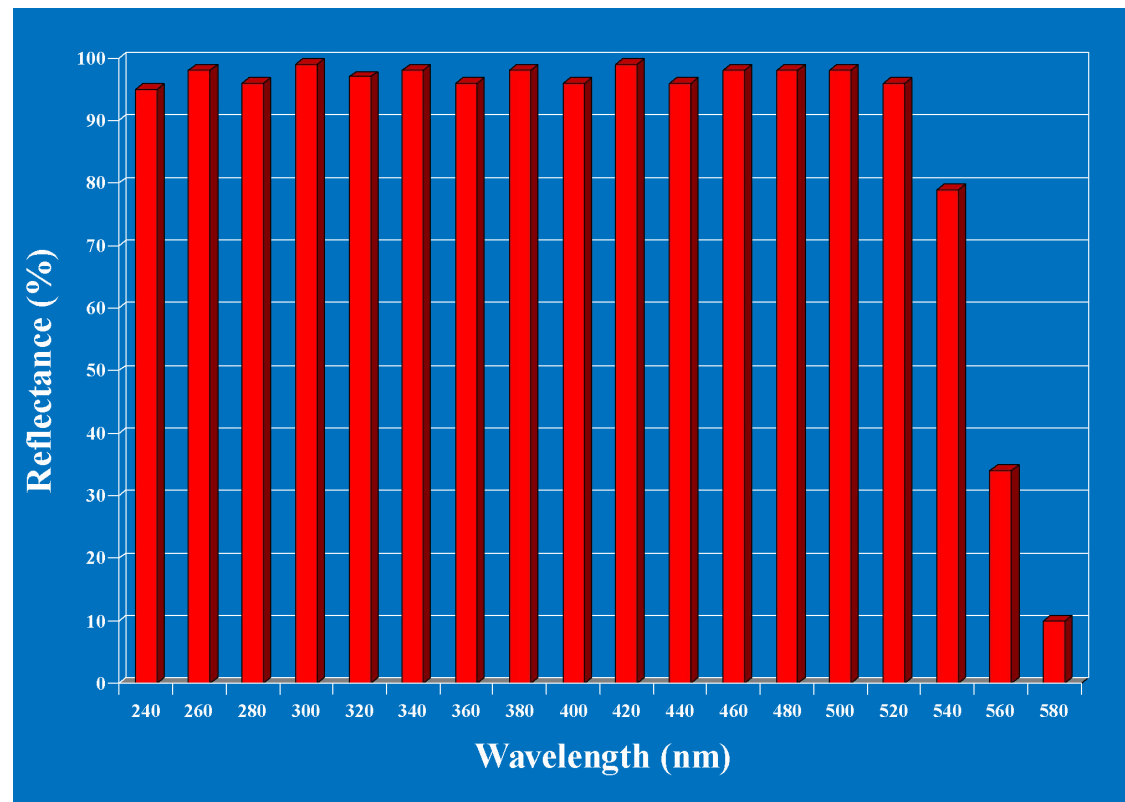
高达 90% UV波段的反射率
